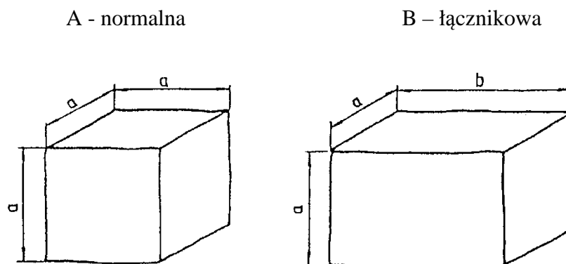
Rysunek 1. Kształt kostki regularnej normalnej i łącznikowej
