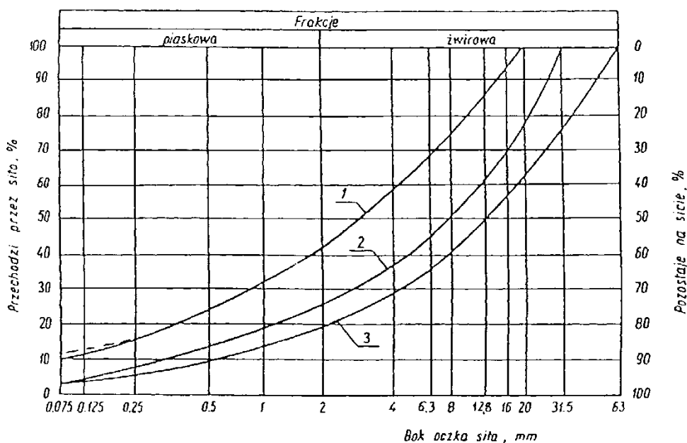
Rysunek 1. Pole dobrego uziarnienia kruszyw przeznaczonych na podbudowę wykonywaną metodą stabilizacji mechanicznej 1-2 kruszywo na podbudowę zasadniczą (górną warstwę) lub podbudowę jednowarstwową 1-3 kruszywo na podbudowę pomocniczą (dolną warstwę)
